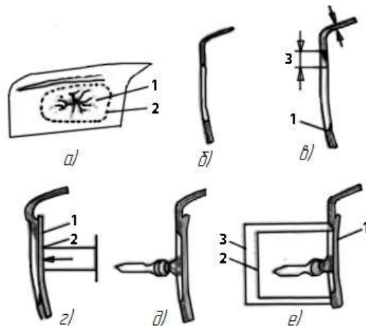
Рис. 6.29. Заделка сквозного повреждения:
