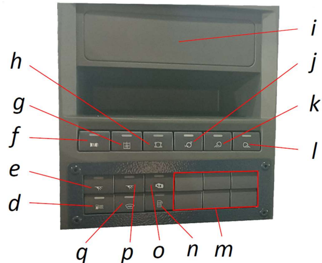
Рис. 5.5 Центральная панель
