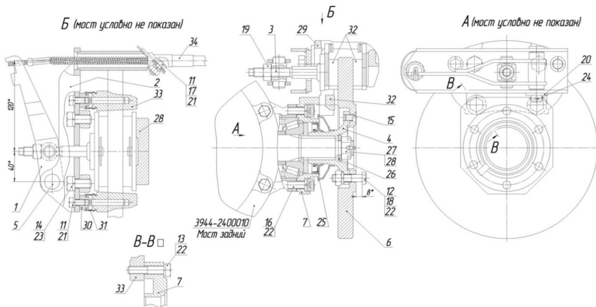
Рис. 6.26 Устройство стояночного тормоза
