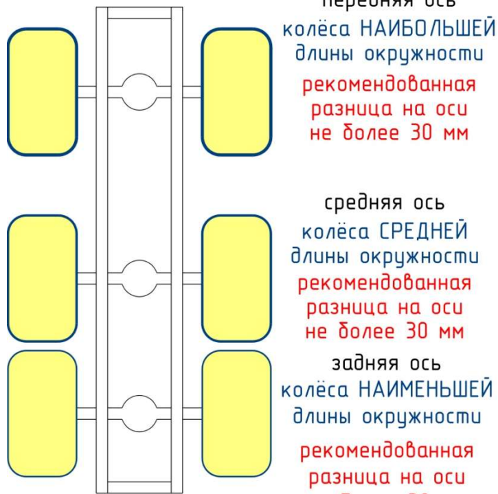
Рис. 10.1 Расстановка колёс
