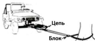
Рис. 20.7 В основном то же, что на рис. 20.6. Цепь с распределителем помогает равномерно распределить нагрузку по составным частям автомобиля
