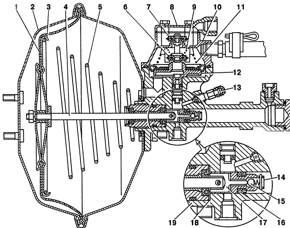
Рис. 6.25 Гидروвакуумный усилитель
