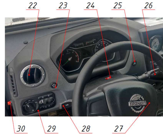
Рис. 5.8 Приборная панель
