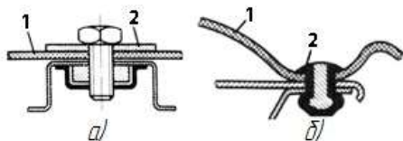
Рис. 6.31. Соединение слоистый пластик-слоистый пластик:
