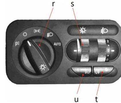
Рис. 5.12 Модуль управления светотехникой (вариант 1)
